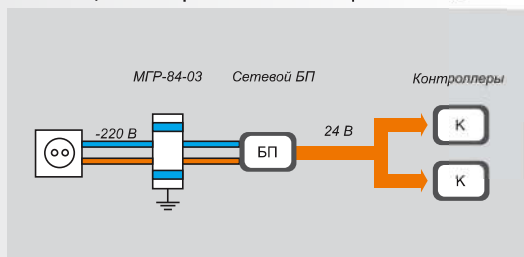
защита от перенапряжений и фильтрация помех в линии ~220 В
