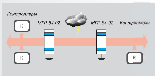
защита магистральной CAN большой протяженности
