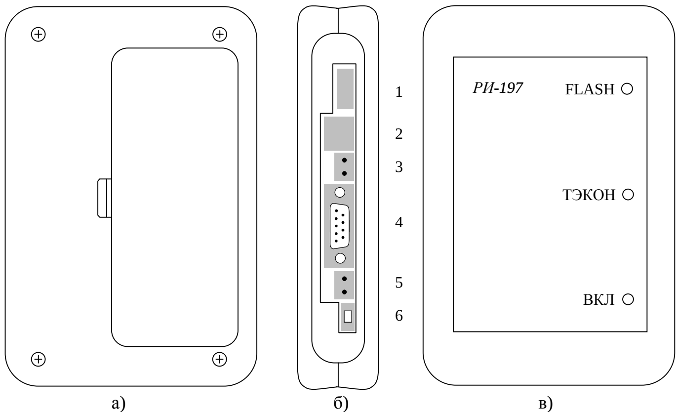
Рисунок 1.1 – внешний вид регистратора
