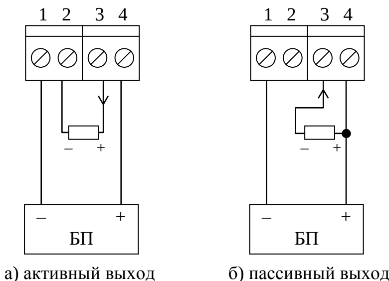
Рисунок 3.4 – схема подключения генераторов тока (номера клемм для ГТ1, измеритель тока изображен как резистор, направление тока указано стрелкой)
