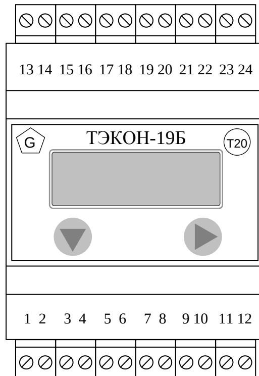
Рисунок 2.1 – Внешний вид передней панели и нумерация клемм ТЭКОН-19Б
