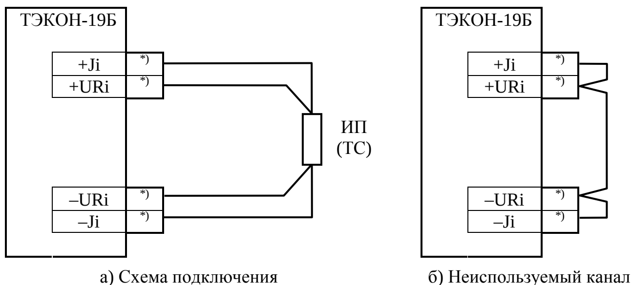
Рисунок 3.1 – Схема подключения измерительных преобразователей температуры типа ТСМ, ТСР
