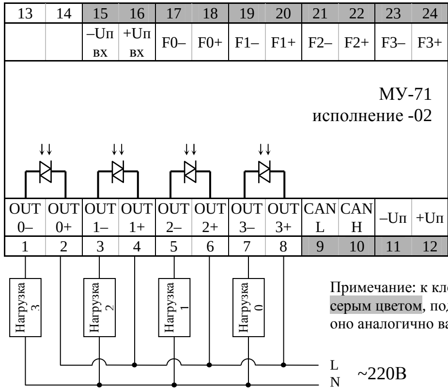
Рисунок 3.1 – Схемы подключения МУ а) исполнение -01; б) исполнение -02
