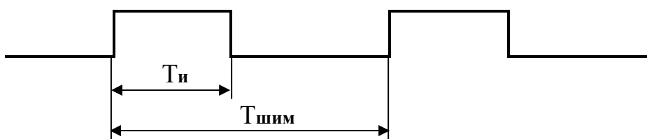
Рисунок 2.2 – сигнал ШИМ
