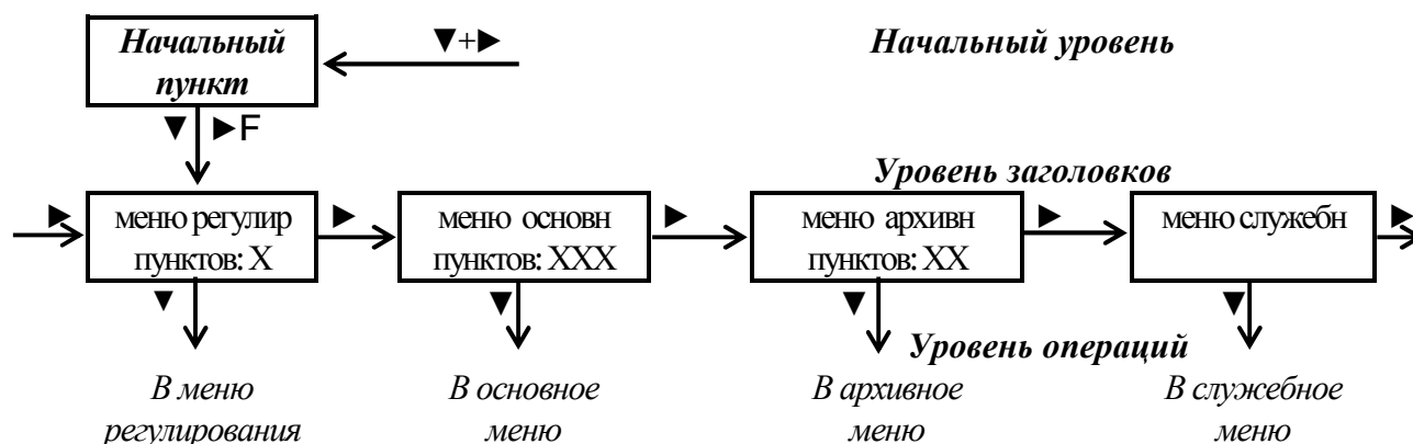
Рисунок 2.7 - Общая структура меню
