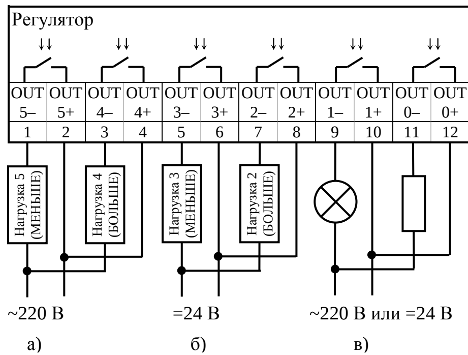
Рисунок 3.4 – Схема подключения нагрузок к выходам регулятора а) исполнительный механизм переменного тока; } работа по принципу б) исполнительный механизм постоянного тока; } «БОЛЬШЕ/МЕНЬШЕ» в) другие исполнительные устройства, с работой по принципу «ВКЛ/ВЫКЛ»
